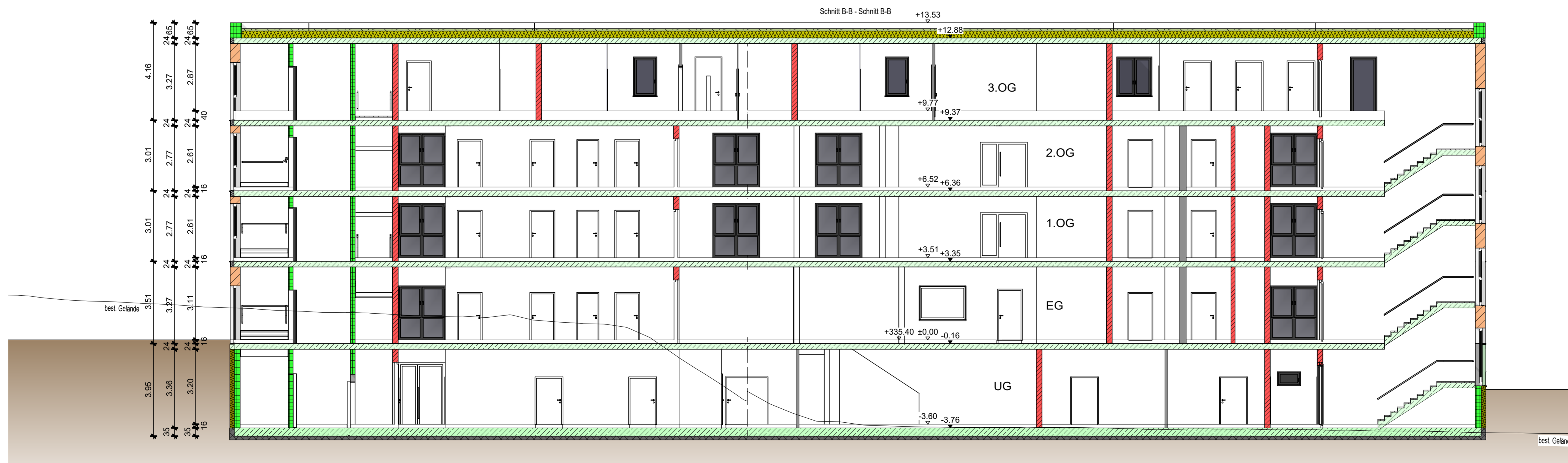
Schnitt B-B - Schnitt B-B
